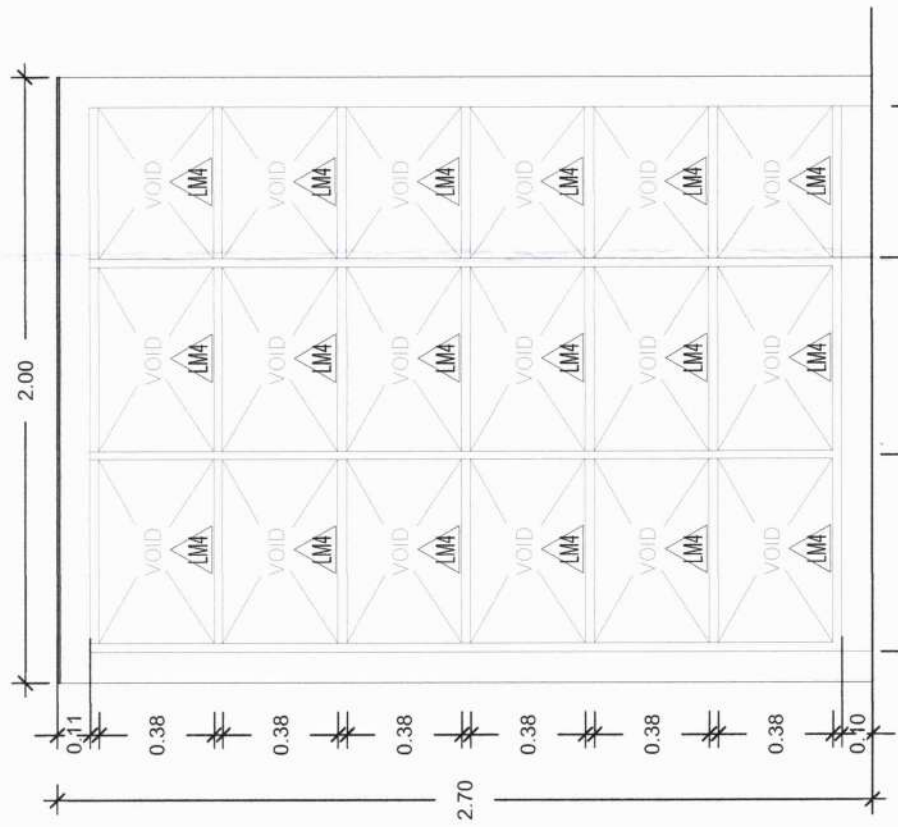
แบบขยายแปลนตู้บิวอิน BSC.no.4 มาตราส่วน 1 : 25
