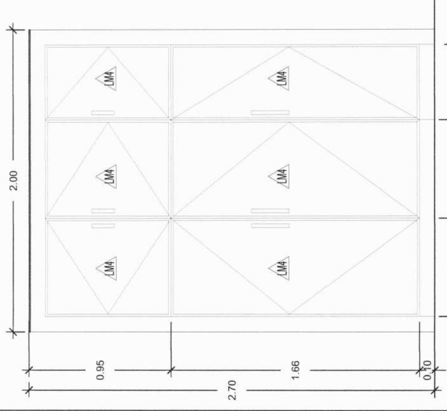
แบบขยายรูปตัด A ตู้บิวอิน BSC.no.4 มาตราส่วน 1 : 25
