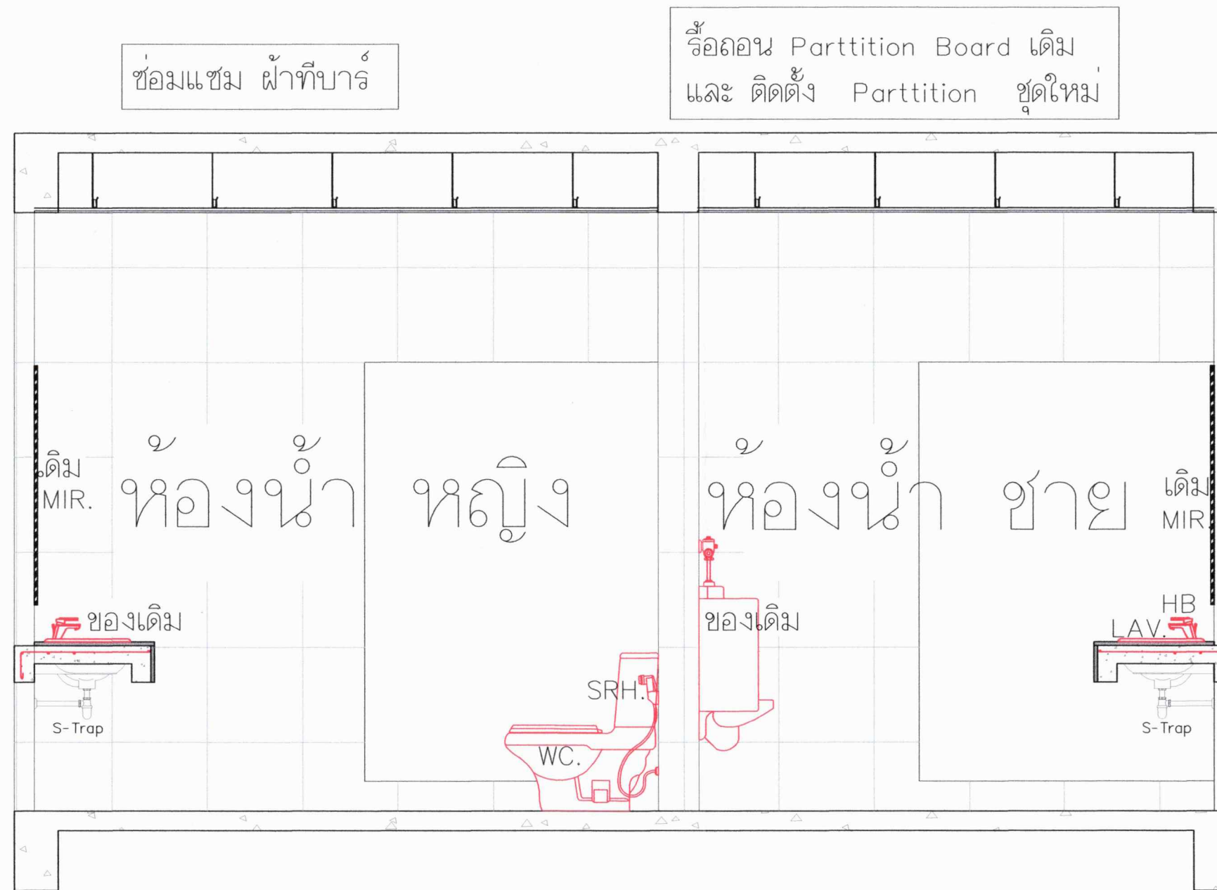
รูปตัดขยายห้องน้ำ/ ญ ชั้น 1 หน้า ER Scale
