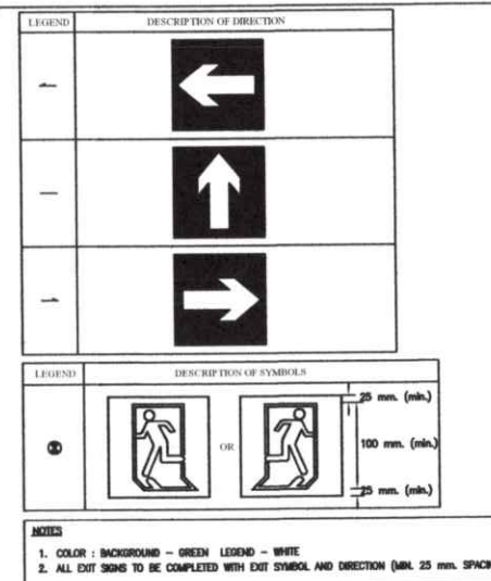
11 EXIT SIGN DETAIL N.T.S.
