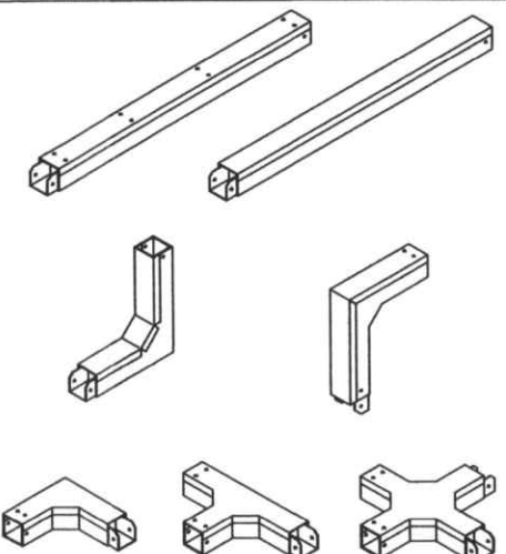
11 WIREWAY N.T.S.
